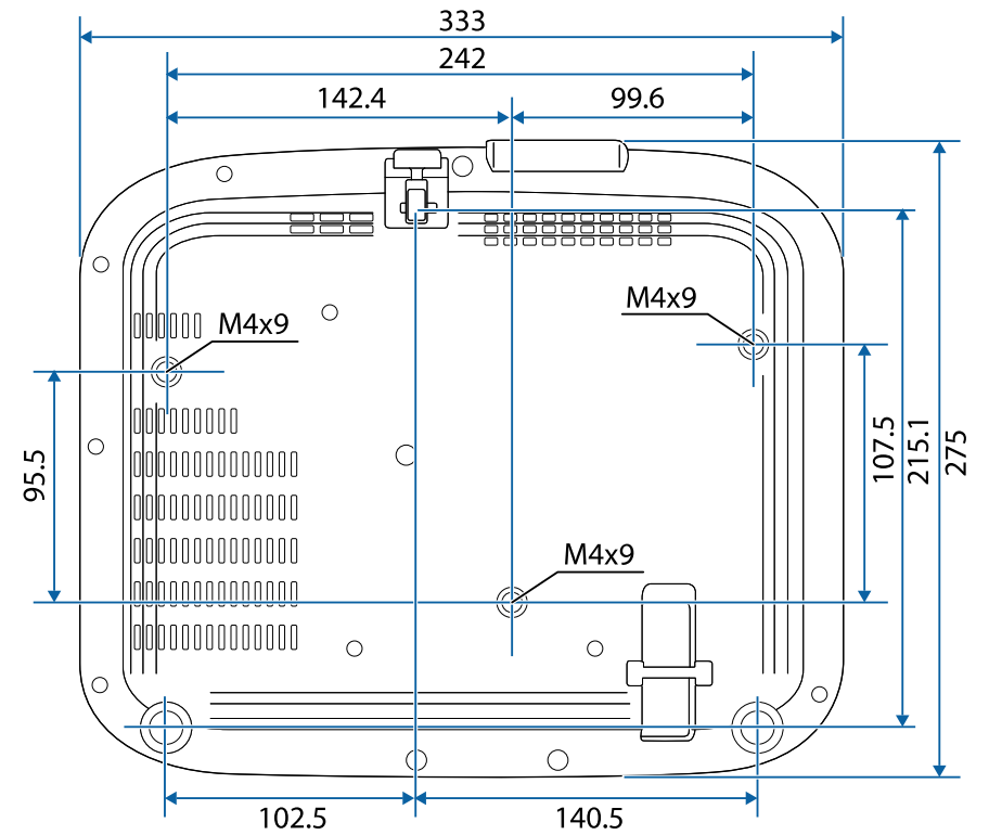
2 Distanța de la centrul lentilelor la punctul de fixare a consolei de suspendare
